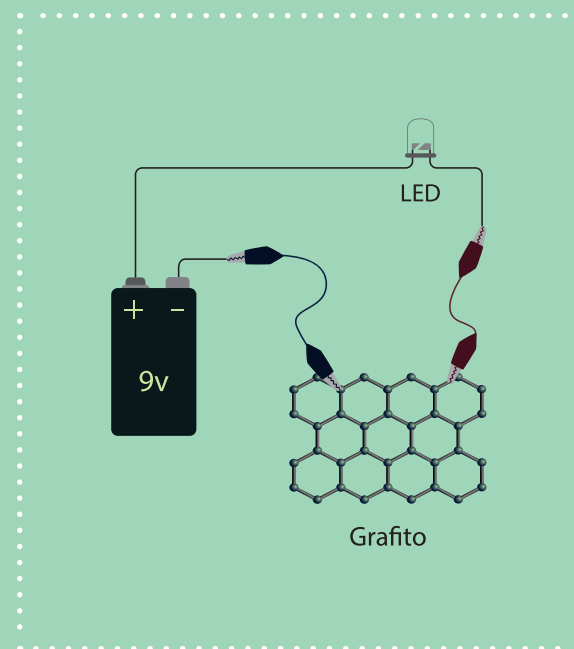
Esquema circuito
